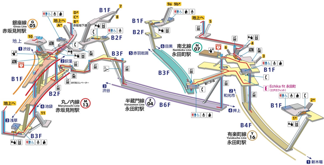
赤坂見附/永田駅構内立体図
